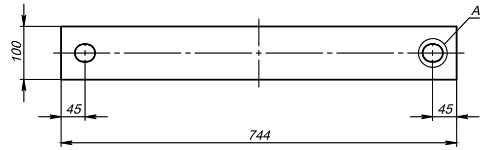
Поз.1 (Полухомут) развертка
