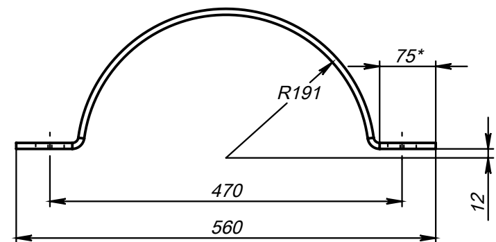
Поз.1 (Полухомут)
